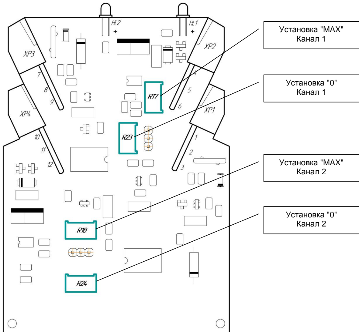
Рисунок 4.1 – Схема расположения элементов настройки БПГ-422
