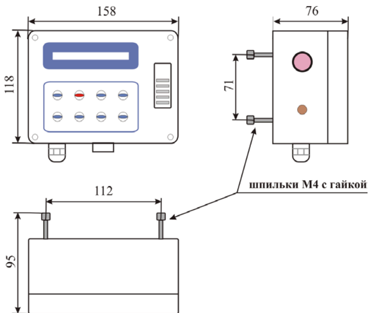
БАУ-ТП-5 - ПДК - габариты
