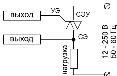
Рис.2. Схема подключения симисторов TC122-25, TC142-80.
